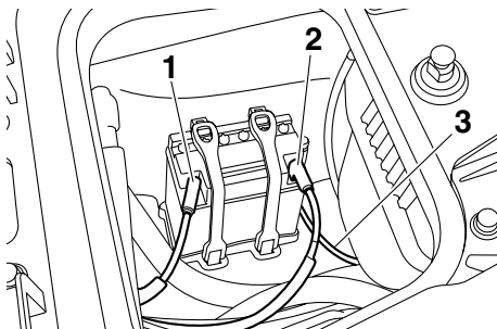
1 Terminal negativo de la batería (-): cable negro
