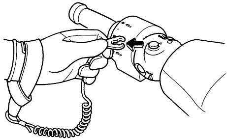
3 Interruptor de paro de emergencia del motor
