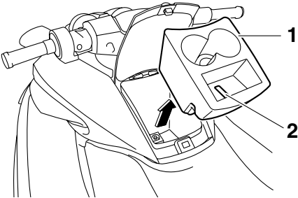
1 Portabebidas 2 Soporte del transmisor
