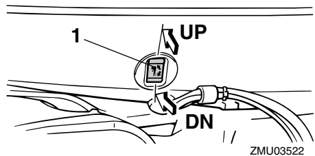
1. Interruptor de elevación y trimado del motor
