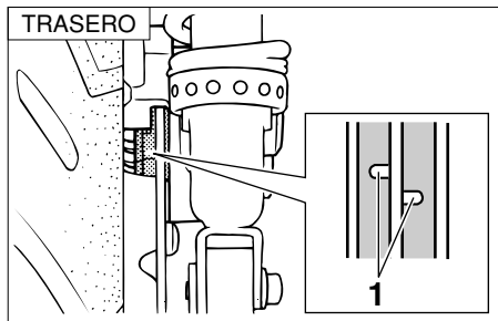
1. Ranura indicadora de desgaste (×2)
