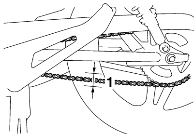
1. Antriebsketten-Durchhang
