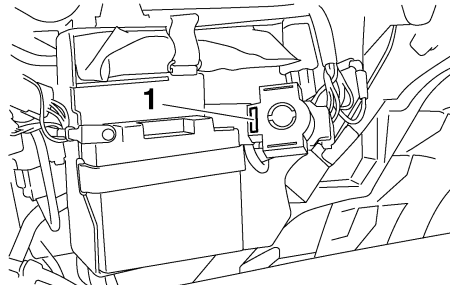
1. Ersatzsicherung
