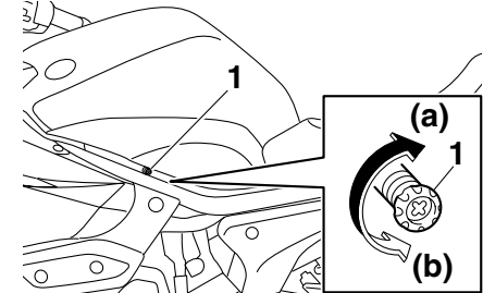
1. Tornillo de ajuste del ralentí
