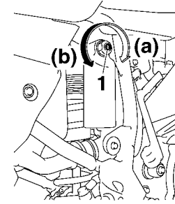
1. Vis de réglage de la force d'amortissement à la compression
