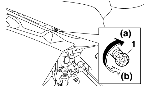
1. Tornillo de ajuste del ralenti
