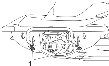
1 Tapón de achique de popa
