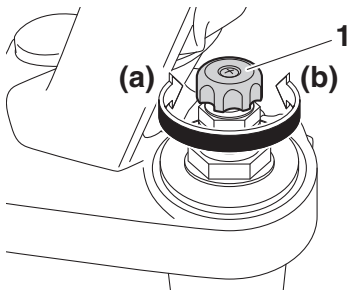
1. Regulador hidráulico del hidráulico de extensión
