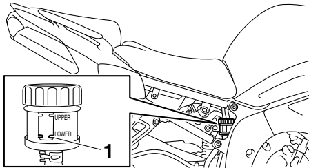
1. Minimalstand-Markierung
