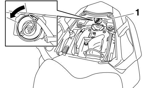
1. Douille d'ampoule de feu arrière/stop
