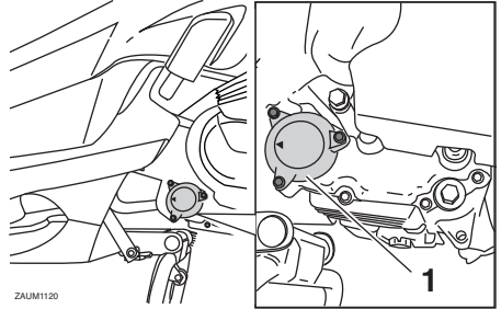
1. Cobertura do elemento do filtro de óleo
