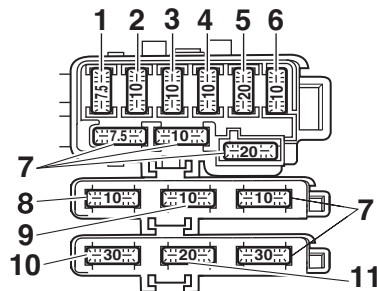
1. Scatola fusibili
