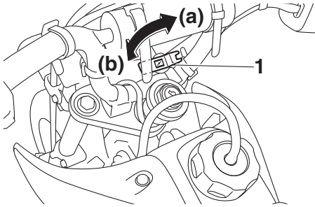
1. Chokehebel “|”
