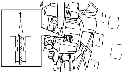
1. Ergot d'indication d'usure de plaquette de frein
