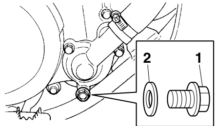
1. Vis de vidange du liquide de refroidissement 2. Joint
