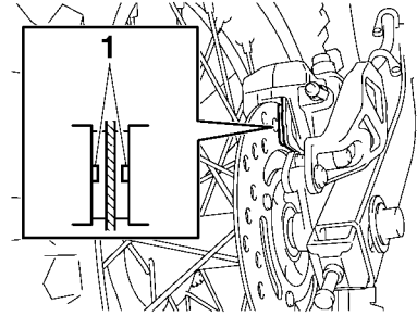
1. Rainure d'indication d'usure de plaquette de frein
