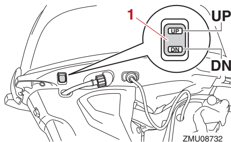
1. Interruptor de elevación del motor
