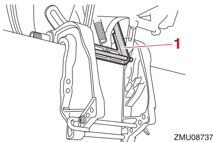
1. Barra soporte
