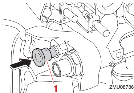
1. Varilla de soporte del motor elevado
