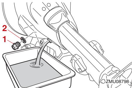
1. Tornillo de drenaje 2. Junta
