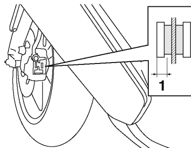
1. Espesor del forro
