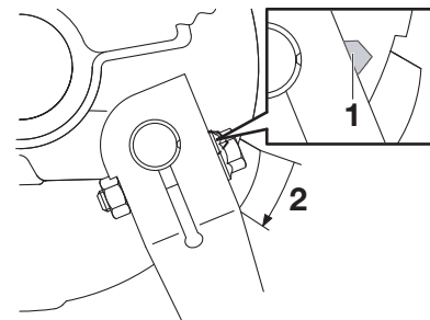
1. Indicador de desgaste 2. Línea de límite de desgaste
